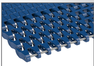
Design aggiornato della catena MatTop serie 1275-1285 Rexnord – modulo esterno
