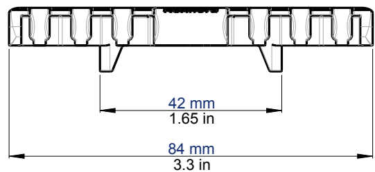
Rexnord-MatTop-Kette der Serie 1001-84mm – Vorderansicht
